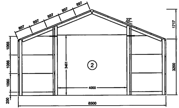
3 REAR ELEVATION SCALE: 1:75
