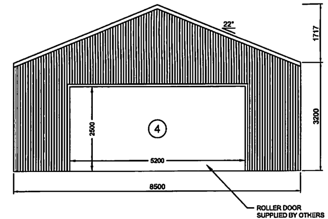
3 REAR ELEVATION SCALE: 1:75
