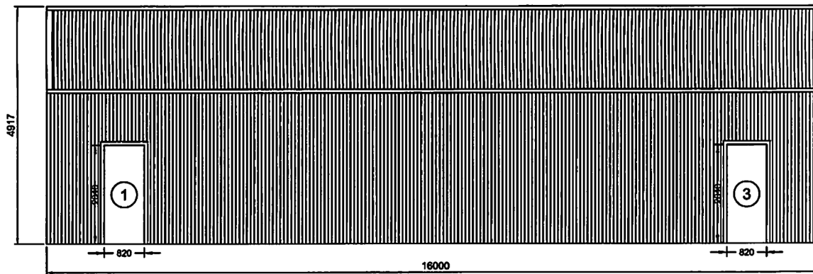
2 LEFT ELEVATION SCALE: 1:75
